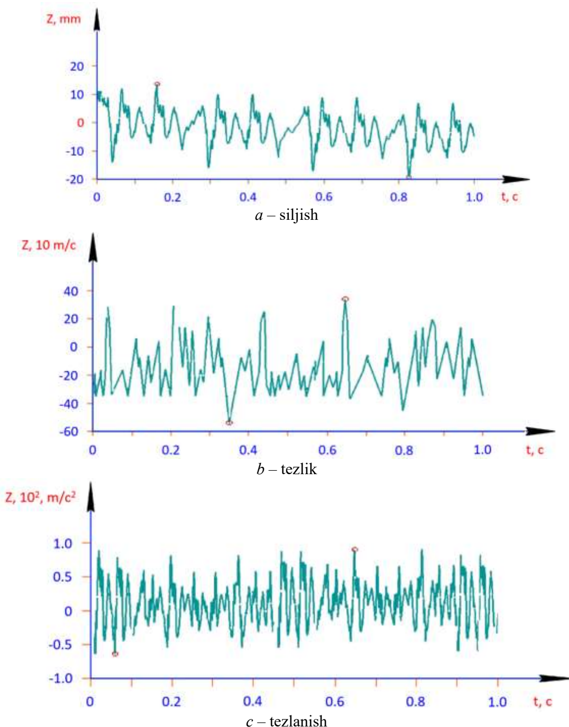
3 - rasm. Tasmali konveyer podshipnik tayanchi qayishqoq vtulkadan tashkil topgan rolikli mexanizmlari oqining vertikal siljish, tezlik va tezlanishdagi tebranishlarini o'zgarish qonuniyatlari.
