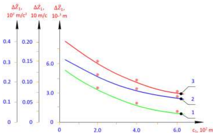
4 - rasm. Tasmali konveyer podshipnik tayanchi qayishqoq vtulkadan tashkil topgan rolikli mexanizimlarining siljish, tezlik, tezlanish qamrovlarini kirish podshipnigi rezina vtulkasini bikirlik koeffitsiyentiga bog'liqlik grafigi.
